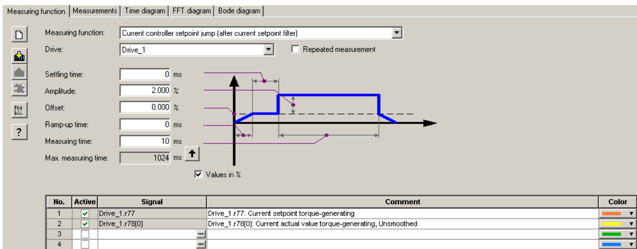
图 4-10 “测量功能”初始画面
