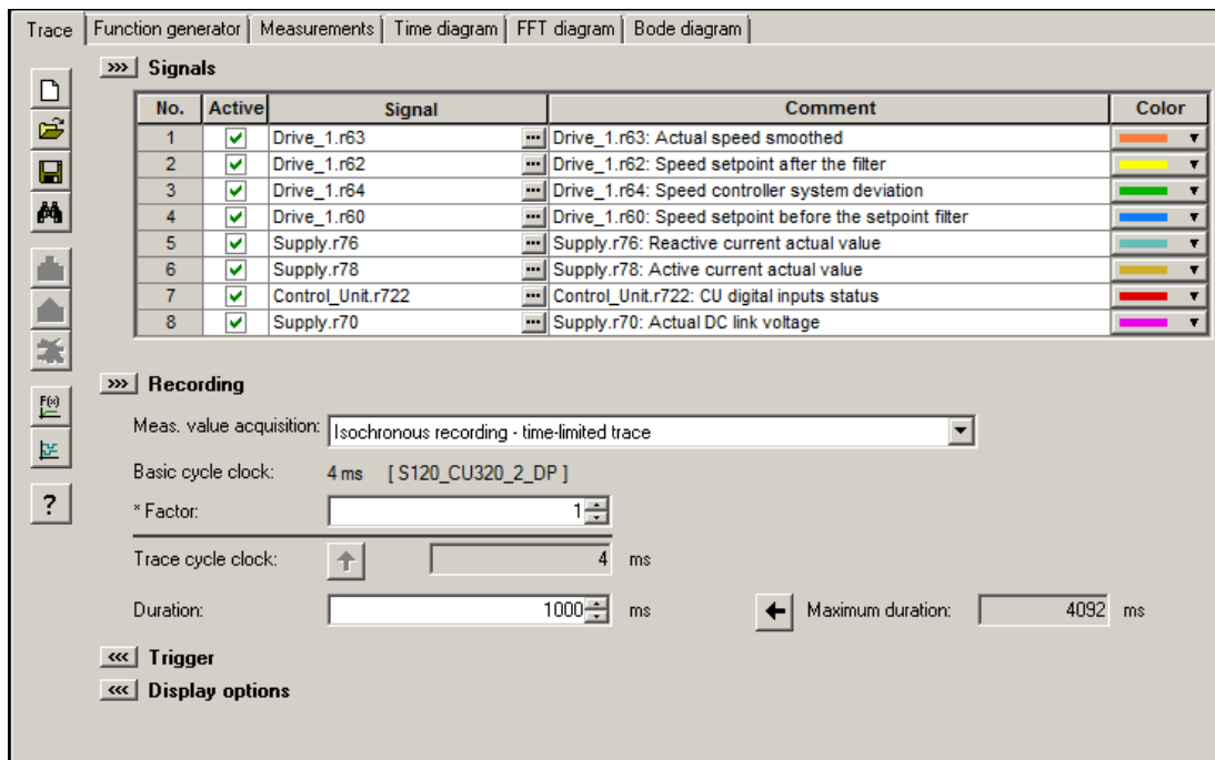
图 4-4 跟踪(Trace)功能
