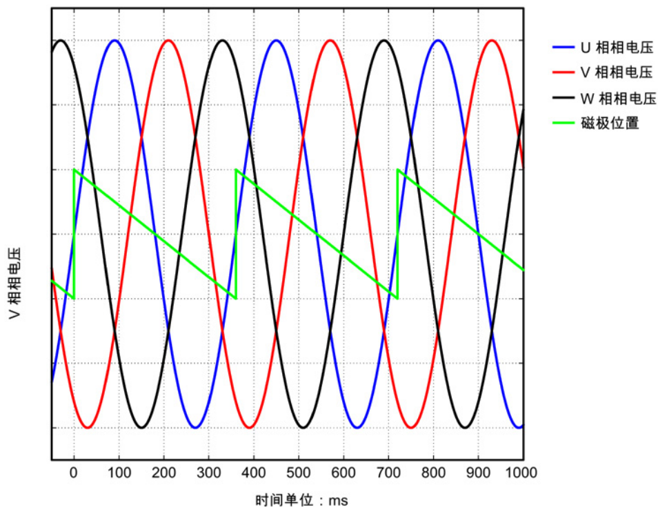
图 3-93 转速实际值取反错误时的 EMF
