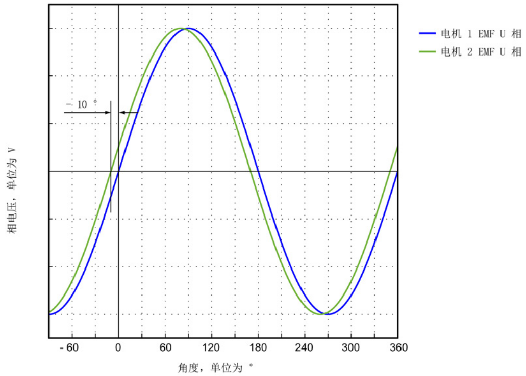
图 3-87 电机 1 的 U 相允许最多滞后电机 2 的 U 相 10°
