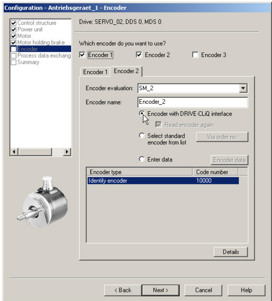
图 3-37 识别 DRIVE-CLiQ 编码器
