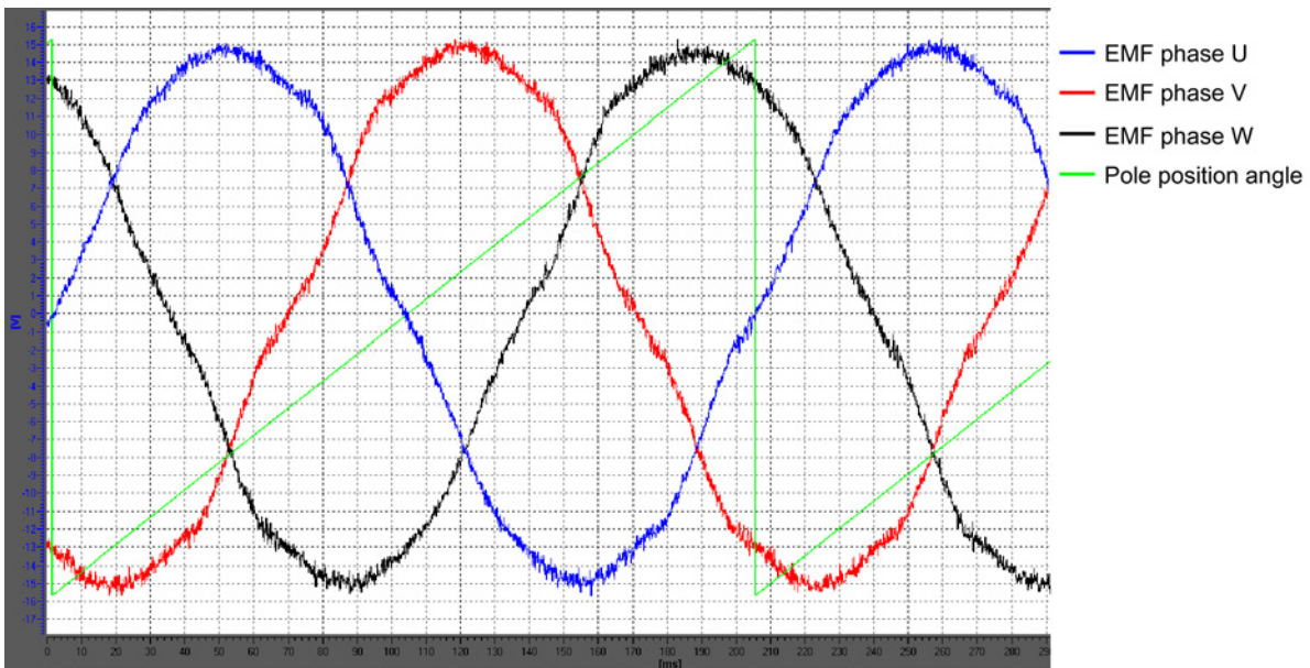
图 3-92 达到最佳换向状态的电机示例（使用调试工具 STARTER 的跟踪功能进行记录）
