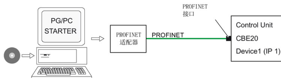
图 3-19 通过 PROFINET 将 PG/PC 和目标设备连接在一起 (示例)
