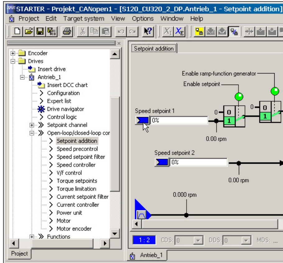
图 3-7 设定值相加
