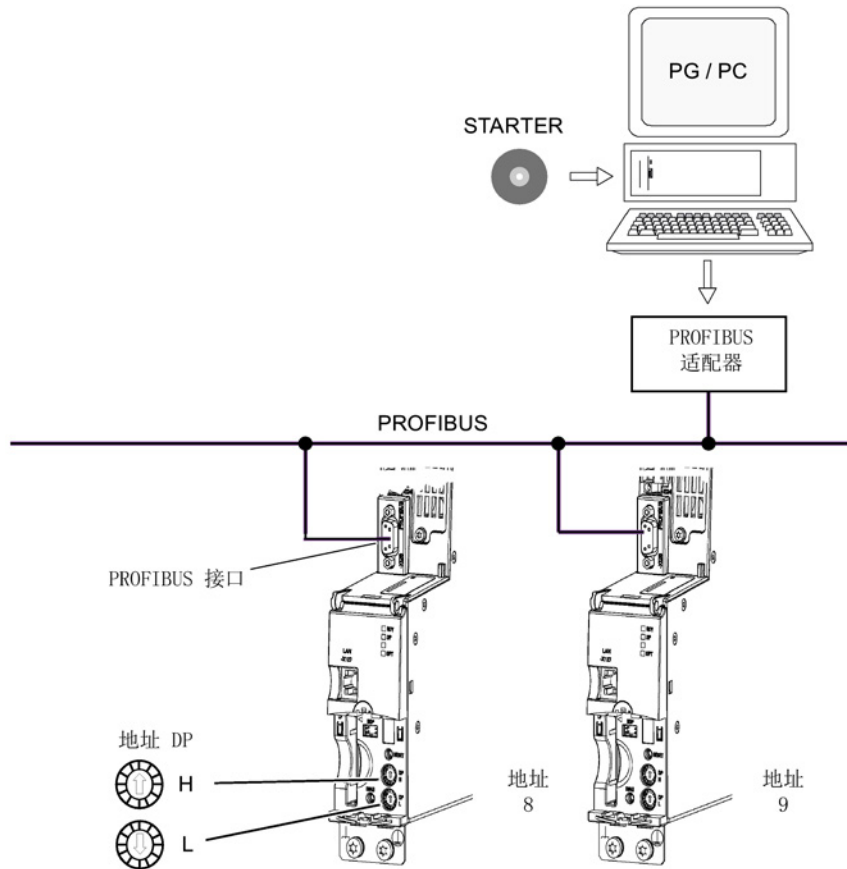
图 3-13 通过 PROFIBUS 将 PG/PC 和目标设备连接在一起
