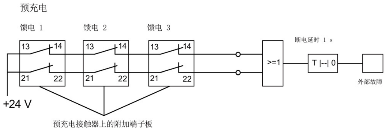
图 3-36 预充电接触器监控
