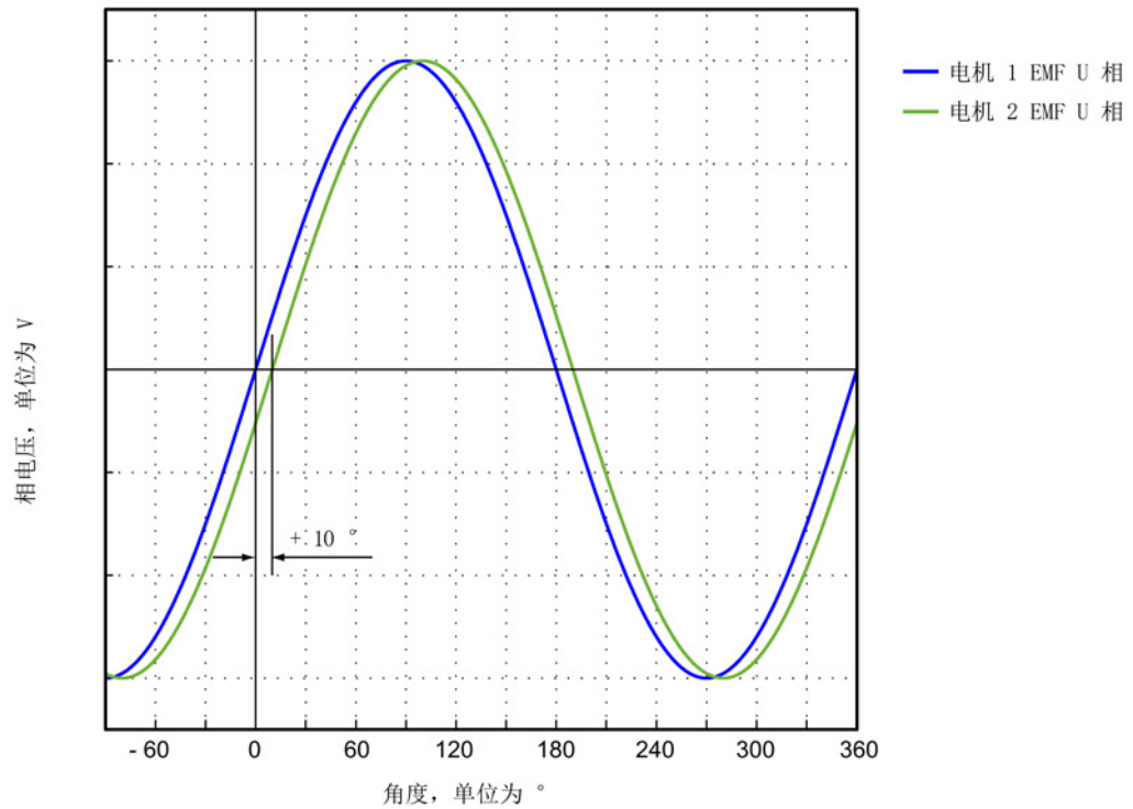
图 3-88 电机 1 的 U 相允许最多提前电机 2 的 U 相 10°
