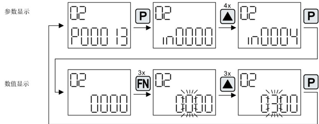
图 3-102 示例：将 p0013[4] 从 0 修改到 300
