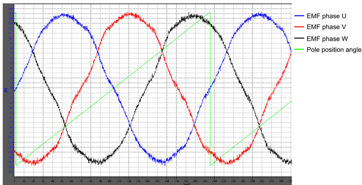
图 3-63 达到最佳换向状态的电机示例（使用调试工具 STARTER 的跟踪功能进行记录）
