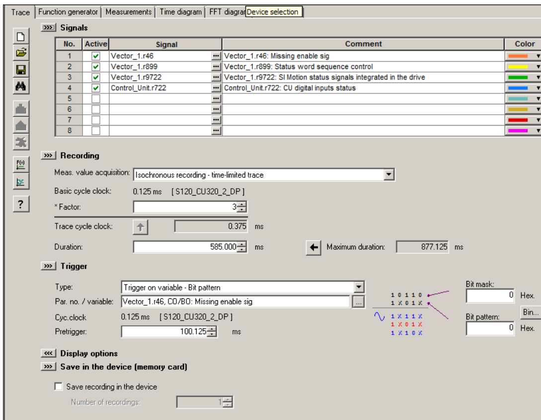
图 4-6 STARTER 中的多次跟踪
