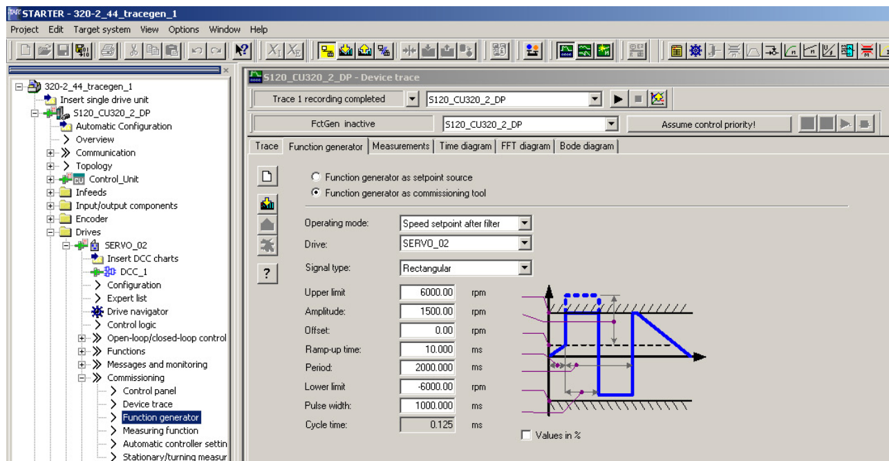
图 4-3 函数发生器
